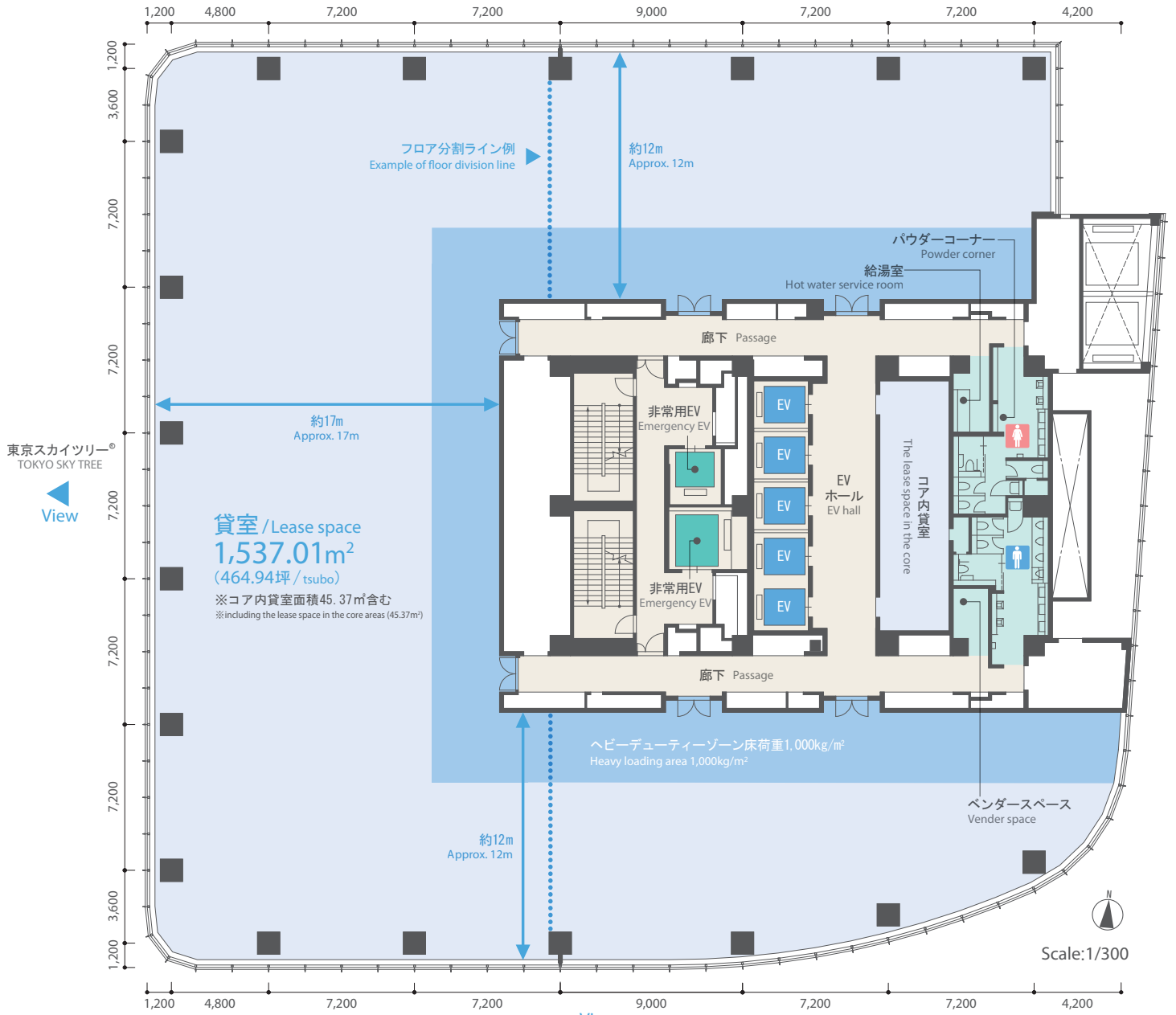
基準階平面図 (26F~29F) Standard floor plan (26F-29F)
